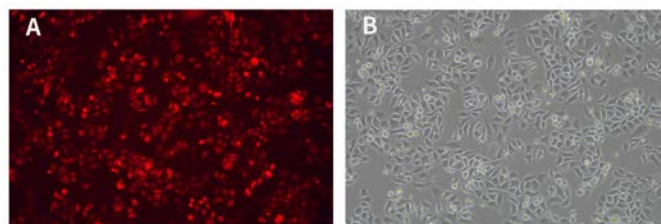
图1. 碧云天IL-6 promoter-Luc-EF1 \alpha -mCherry HeLa Cells (C8551) 的荧光显微镜观察图。A为荧光照片, B为明场照片。实际检测效果会因检测仪器、实验条件的不同而存在差异, 本图仅供参考。
